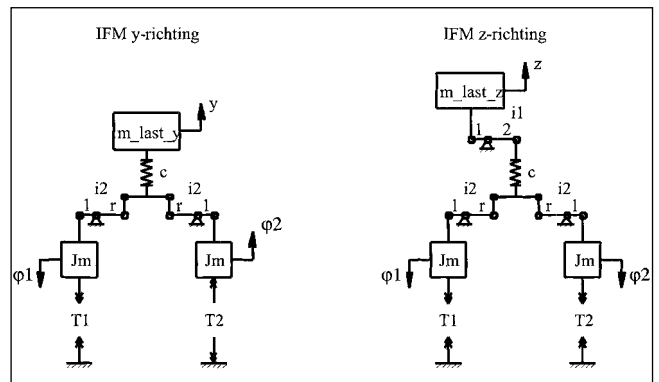
Figuur 2. Ideaal Fysisch Model Pick-and-place unit.
