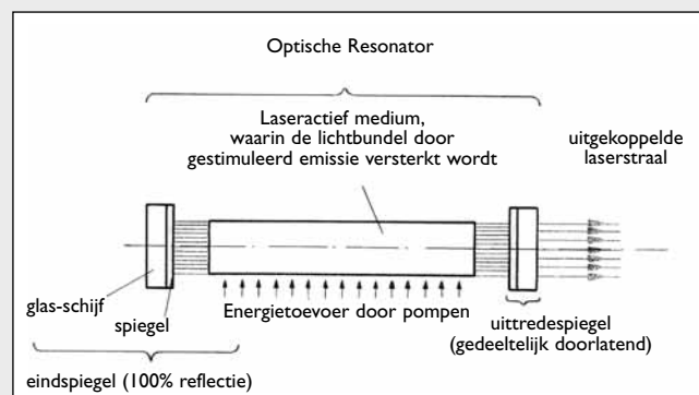
Figuur I/1. De drie basiselementen van elke laser: het laserende materiaal, de pompbron en de trillholte.
