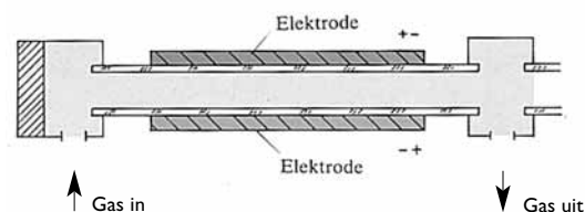
Figuur 4. Twee voorkomende principes van ontladingssystemen bij CO 2 lasers. Boven een hoogspanning DC-uitvoering: beide elektroden in rondstromend lasergas. Onder de fraaiere hf-constructie met gedeelde metalen mantelelektrode buiten om de glazen laserbuis.
