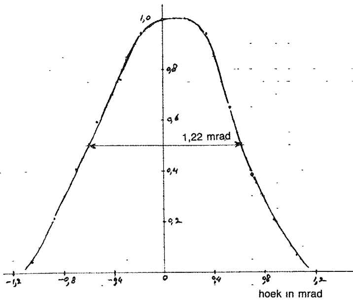
figuur 6 Verticale "point-spread-function" voor de 10 \mu\text{m} spectrale band
