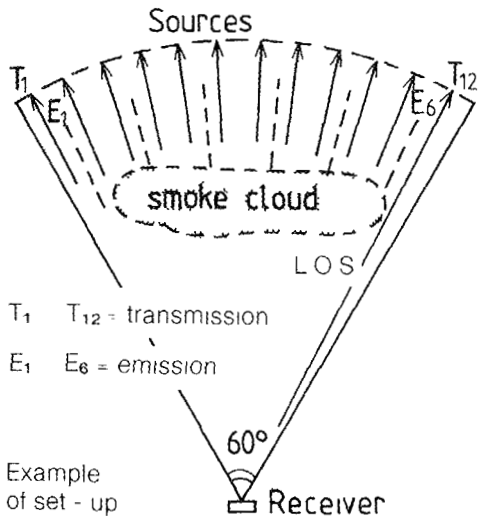
figuur 2 Illustratie van de opzet van de transmissio-radiometer
