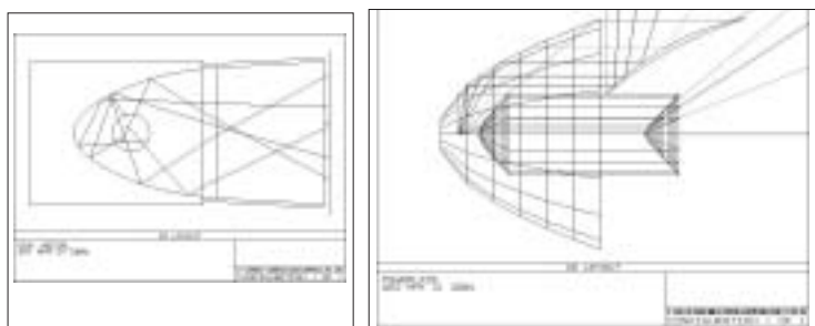
3D-simulaties van IPL-lens en -reflector (links) en van non-imaging optiek met power-LED.
